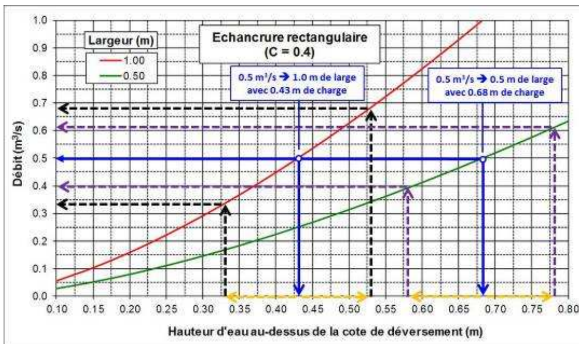
Figure 7 : Illustration des variations de débit suite à des variations de niveau d'eau de +/- 10 cm, pour des échantures rectangulaires dénoyées de 0.5 m et 1.0 m de large, calées pour 0.5 m³/s.
