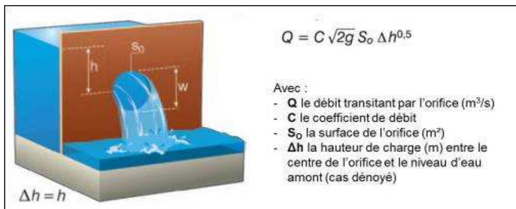
Figure 11 : Formule pour le calcul du débit transitant par un orifice dénoyé (figure adaptée de Le Coz et al. 2011).
